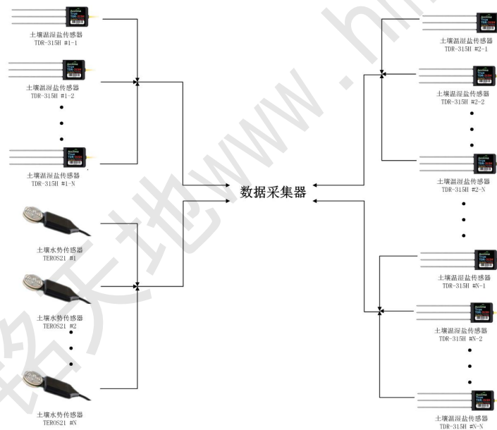
图 1 矩阵式土壤温湿盐系统结构示意图
